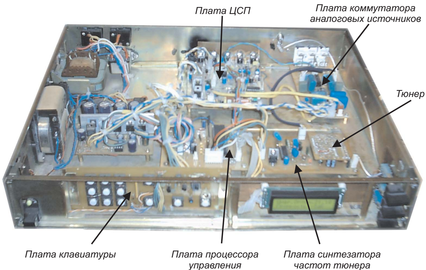
Внешний вид ресивера в корпусе от эквалайзера "Феникс-008"
